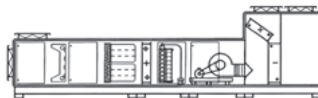
Unità trattamento aria tipo multizone.
